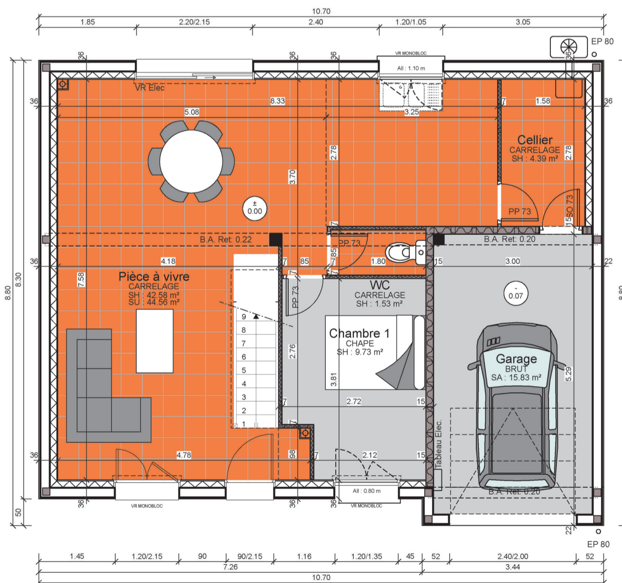
Maison ARAL 4.099 GI Plan du rez-de-chaussée
