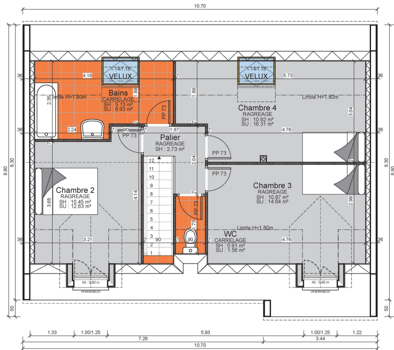
Maison ARAL 4.099 GI Plan de l'étage
